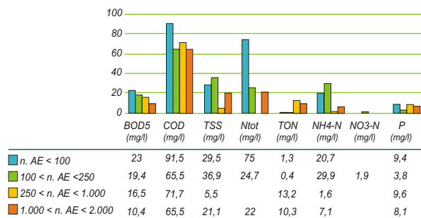
Sistemas con flujo sumergido horizontal como tratamiento secundario
