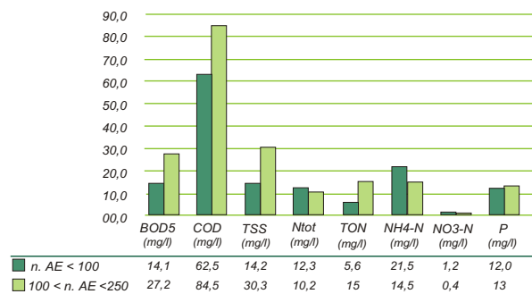
Sistemas con flujo sumergido horizontal como tratamiento secundario
