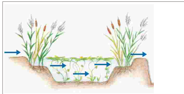
Representación esquemática de un sistema con flujo sumergido horizontal de un sistema con flujo sumergido vertical y representación esquemática de un sistema con flujo libre.
