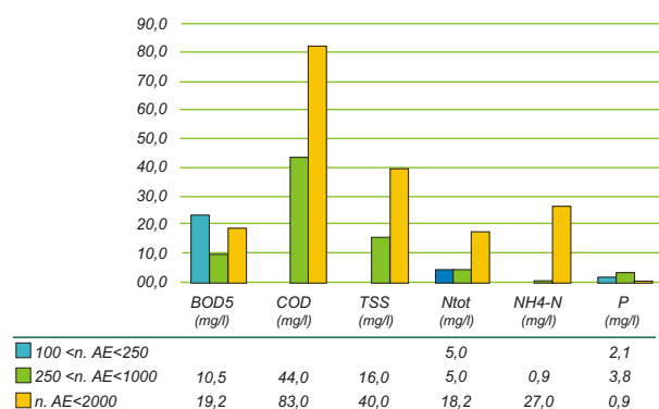
Sistemas con flujo sumergido vertical como tratamiento secundario
